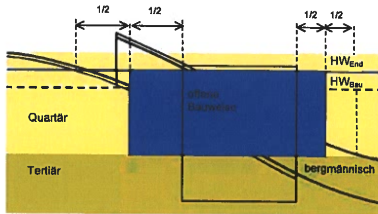
Abb. 10.2: Schemadarstellung: Zur Berechnung angesetzter Baukörper im Grundwasser bei HW_{End}
